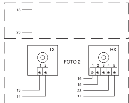
Fig. 3C Conexión fototest con la fotocélula "Fotocélula 2" sola
