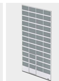
Ворота со сплошным остеклением с перемычкой (ширина проема до 6 100 мм)
